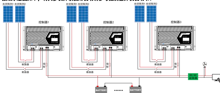
图2-5多机并联接线示意图
