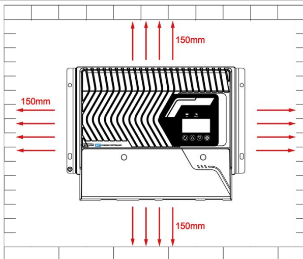
图2-1 安装示意图（IP43）
