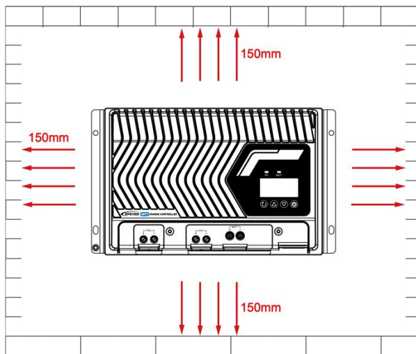
图2-2安装示意图（IP32）
